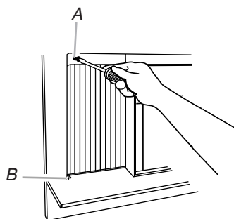
A. Tornillo de cabeza redonda #10 x 3/4" B. Orificio para tornillo de cabeza redonda #10 x 3/4"
