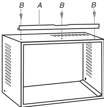
A. Canal superior B. Tornillos Phillips de cabeza de arandela #10 x 3/8" (3)
