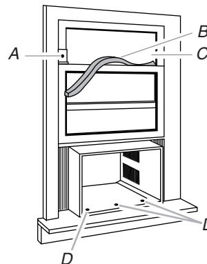
A. Soporte de seguridad de ventana B. Obturador de espuma del marco de la ventana C. Cristal de la ventana superior D. Tornillos Phillips de cabeza de cono achatado #10 x 1/2" (3)
