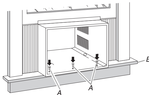
A. Tornillos Phillips de cabeza de cono achatado #10 x 1/2" B. Repisa de la ventana
