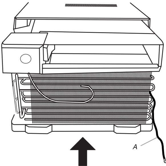
A. Alambre a tierra fuera del gabinete
