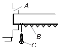
A. Canal de la ventana B. Cortina izquierda C. Tornillo de cabeza redonda #10 x 3/4"
